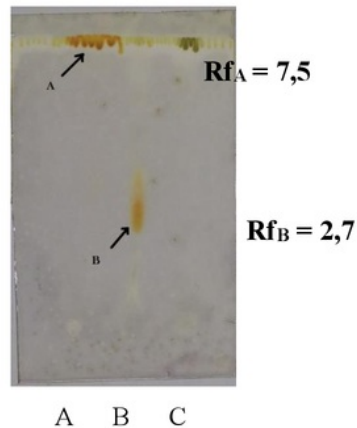
Gambar 2. Hasil uji bebas alkaloid, A (kontrol positif Piper nigrum L), B(noda ekstrak tidak bebas alkaloid), C (ekstrak bebas alkaloid), KLT silika GF 254 nm, diklorometan : metanol (9:1), pereaksi Dragendorff.
