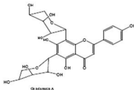
Gambar 1. Struktur gendarusin A
