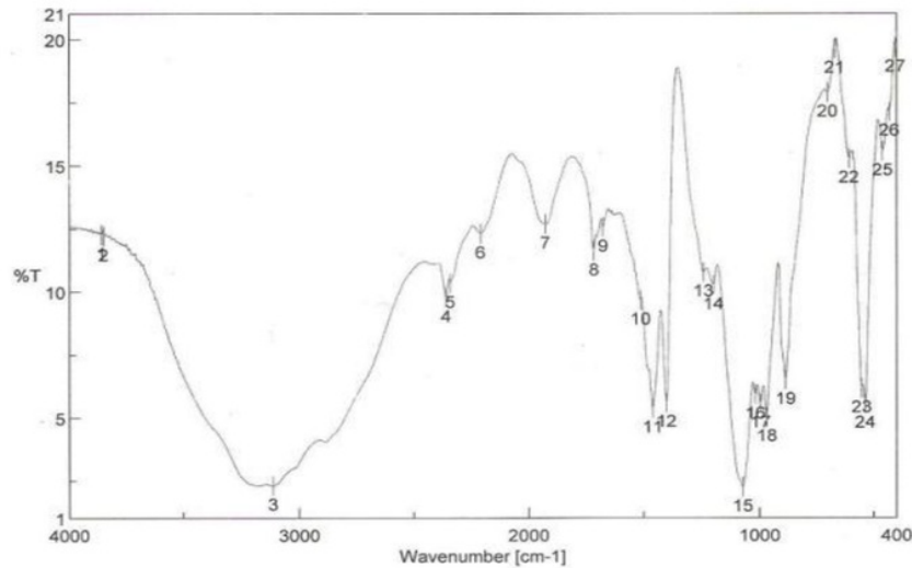
Gambar 3. Spektrum FTIR komposit kolagen – hidroksiapatit
