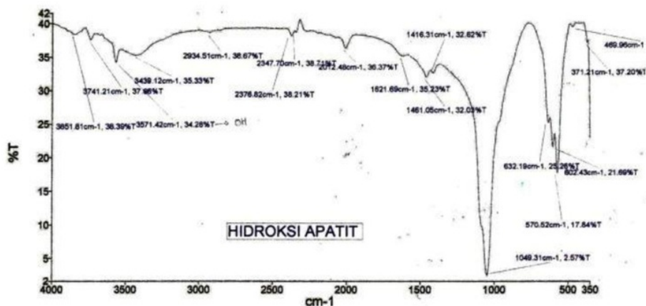
Gambar 2. Spektrum FTIR hidroksiapatit tulang sapi
