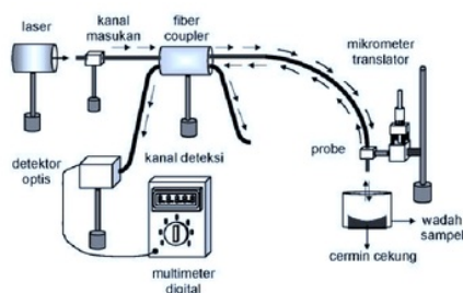
Gambar 2. Set up eksperimen sensor konsentrasi Rhodamin B dalam air.
