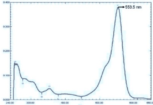
Gambar 3. Spektrum seraban larutan Rhodamine B pada konsentrasi 1 ppm.
