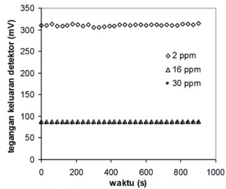
9 Gambar 7. Grafik hasil uji stabilitas sensor.
