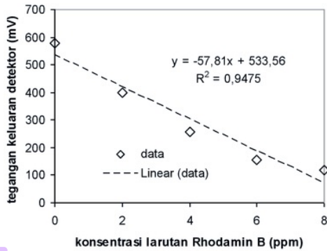
3 Gambar 6. Grafik linier hubungan antara tegangan keluaran detektor terhadap konsentrasi Rhodamin B dalam air.
