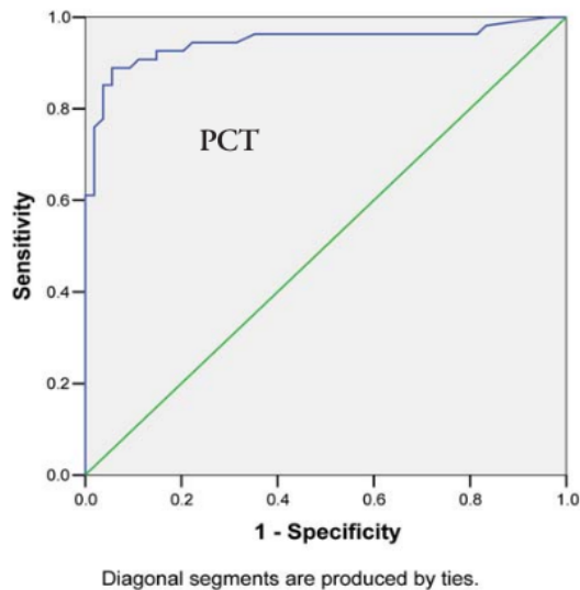
Gambar 1. Kurva ROC akurasi diagnostik kadar PCT Luas area kurva ROC 0,94 ( 0,89 – 0,99 )
