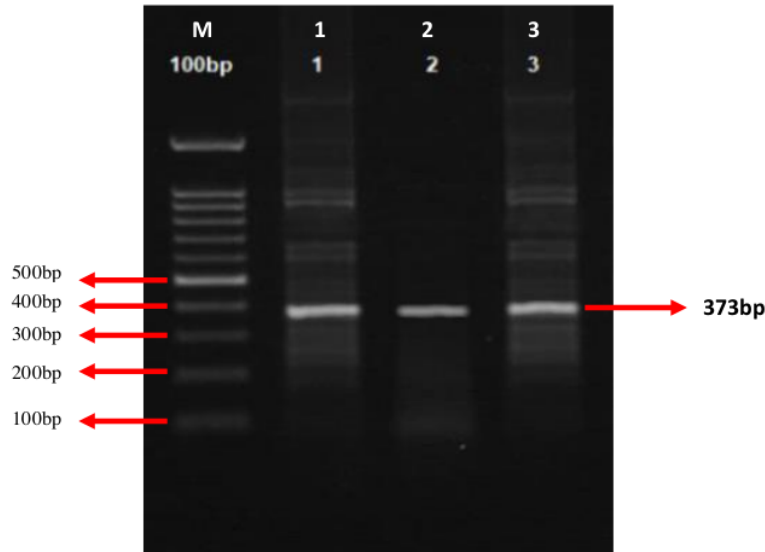
Gambar 1. Hasil elektroforesis PCR pada darah (1) sapi Madrasin, (2) sapi Madura, dan (3) sapi Limousin. Keterangan M=Marker DNA: produk PCR (373 bp).
