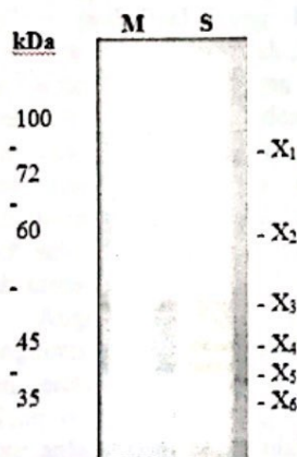
Gambar 2.4. Hasil karakterisasi whole protein spora Myxobolus koi dengan SDS-PAGE menggunakan pewarnaan perak nitrat (Yusuf, 2015).
