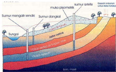
Gambar 5. Kedudukan Tipe Akuifer (Kodoatie, 2012)
