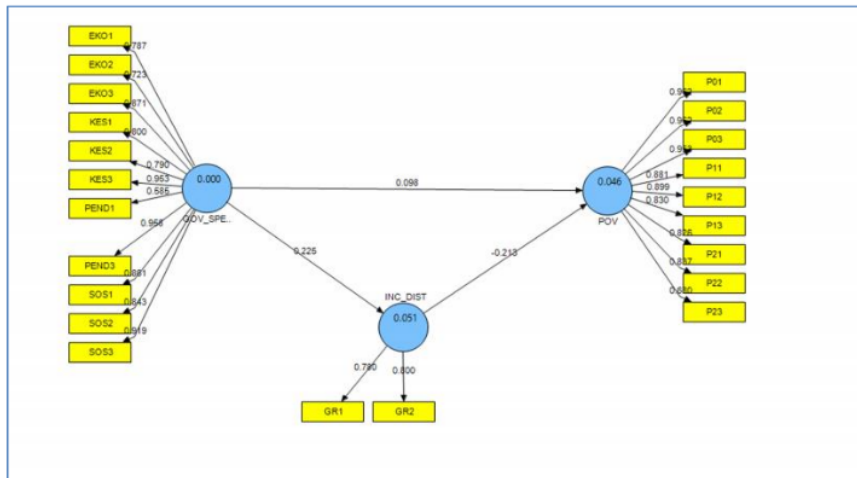
Gambar 5. Diagram Jalur dan Nilai Loading Factor setelah variabel manifest dikeluarkan
