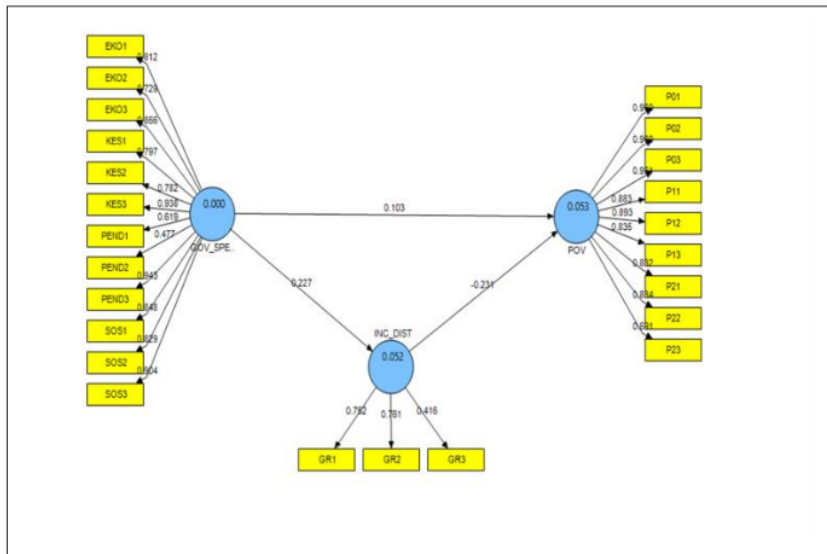
Gambar 4. Diagram Jalur dan Nilai Loading Factor
