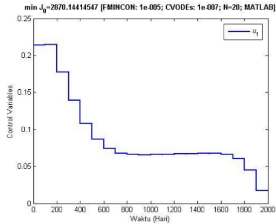
Gambar 6. Grafik Profil Kontrol Upaya Pencegahan ( u_1 )
