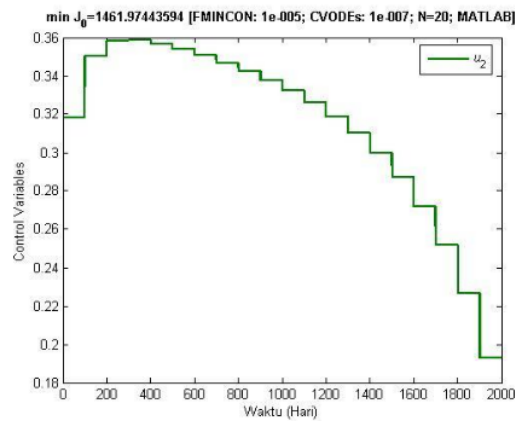
Gambar 7. Grafik Profil Kontrol Upaya Pembasmian ( u_2 )
