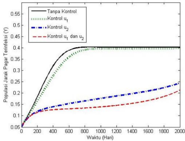
Gambar 4. Simulasi Pemberian Kontrol pada Populasi Jarak Pagar yang Terinfeksi
