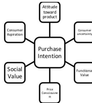
Gambar 1 Kerangka Penelitian
