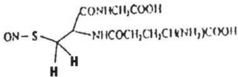
S-Nitrosoglutathione (GSNO)
