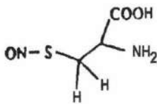
S-Nitroso-L-cystine (CySNO)
