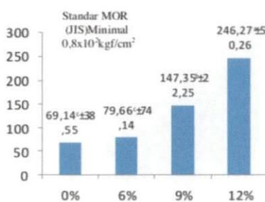
Gambar 6. Grafik keteguhan patah MDF dengan konsentrasi perekat berbeda
