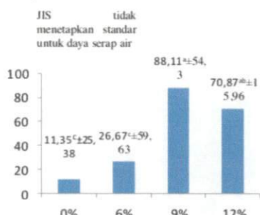
Gambar 3. Grafik daya serap MDF dengan konsentrasi perekat berbeda
