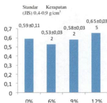
Gambar 1. Grafik kerapatan MDF dengan konsentrasi perekat berbeda
