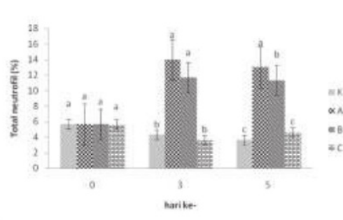
Gambar 2. Diferensial leukosit ikan gurame setelah pemberian ekstrak air panas Spirulina platensis (K= kontrol, A = 1%, B = 10% dan C = 20%)
