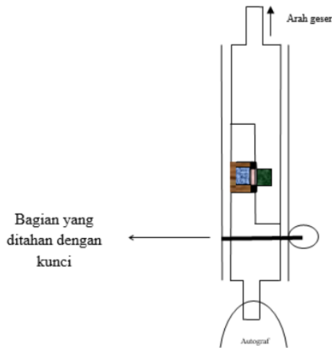
Gambar 1. Alat bantu pengukuran kekuatan geser (plunger)
