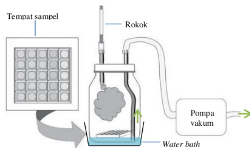
Gambar 1. Smoking machine yang digunakan untuk penelitian. 14
