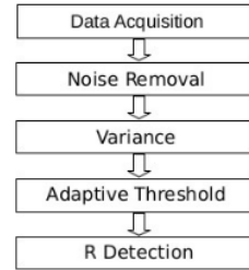
Fig. 2: QVAT methodology
