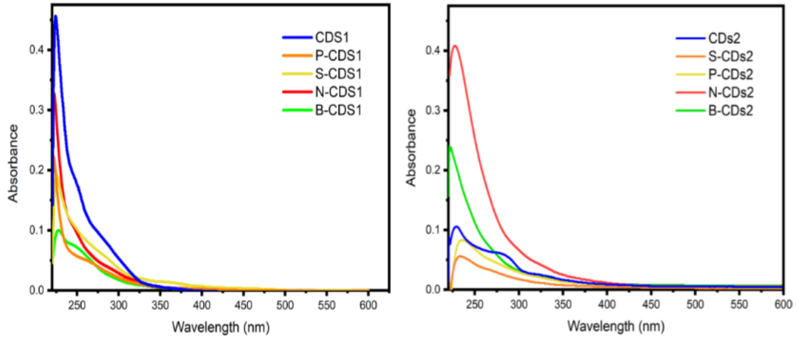
Gambar 1. Spektra UV-Vis karbon dot dengan metode pirolisis dan microwave assisted
