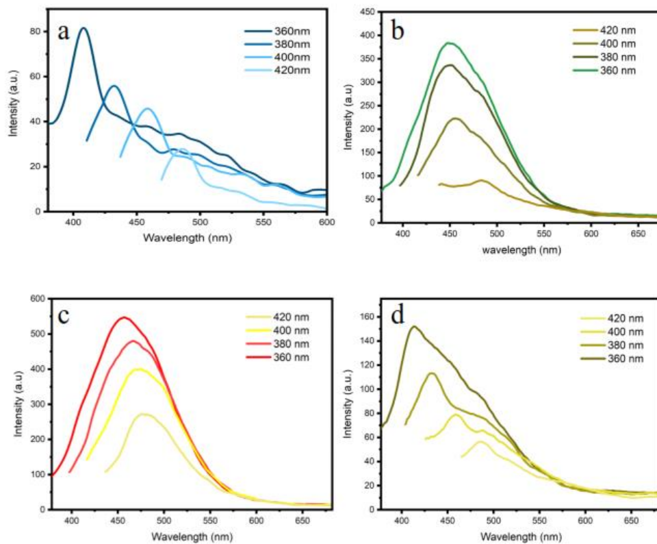
Gambar 3. Spektra photoluminescense (PL) dari a CDs2, b B-CDs2, c N-CDs2, d SCDs2, dan e P-CDs2. F Spektra PL pada Panjang Gelombang eksitasi 360 nm metode microwave-assisted
