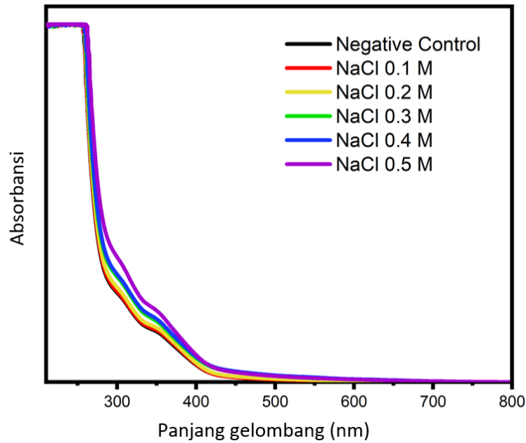
Gambar 15. Spektra UV karbon dot B-CDs2 dengan variasi konsentrasi NaCl
