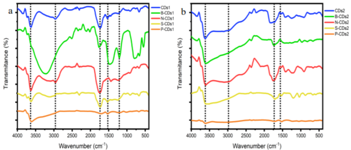
Gambar 5. a Spektra FTIR karbon dot dengan metode pirolisis. b Spektra FTIR karbon dot dengan metode microwave-assisted.
