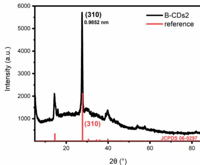
Gambar 6. Difraktogram karbon dot B-CDs2
