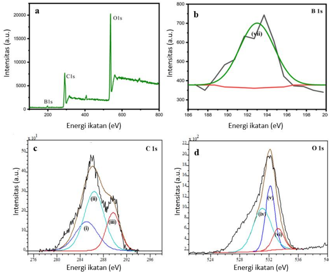
Gambar 7. Spektra XPS Karbon dot B-CDs2 (a) full scan range , (b) spektrum daerah B1s, (c) spektrum daerah C1s, dan (d) spektrum daerah O1s.
