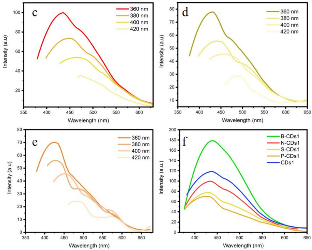
Gambar 2. Spektra photoluminescense (PL) dari a CDs1, b B-CDs1, c N-CDs1, d SCDs1, dan e P-CDs1. F Spektra PL pada Panjang gelombang eksitasi 360 nm metode pirolisis.
