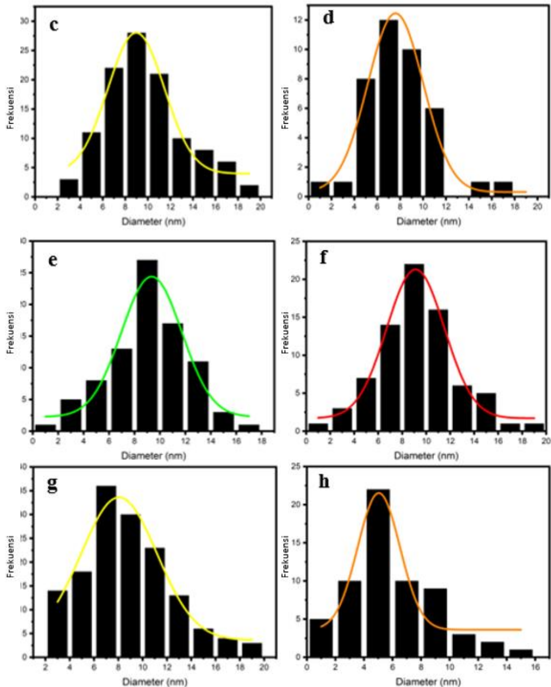
Gambar 9 Histogram distribusi ukuran partikel karbon dot a B-CDs1, b N-CDs1, S-CDs1, d P-CDs, e B-CDs2, f N-CDs2, g S-CDs2, dan h P-CDs2.
