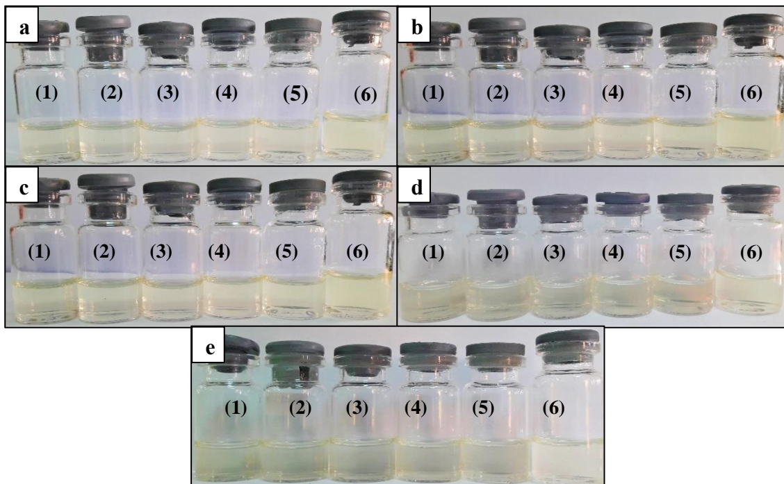
Gambar 14. Uji stabilitas karbon dot B-CDs2 terhadap variasi garam NaCl (1) 0,1 M, (2) 0,2 M, (3) 0,3 M, (4) 0,4 M, (5) 0,5 M, dan (6) tanpa NaCl pada a 0 jam, b 6 jam, c 12 jam, d 24 jam, dan e 7 hari
