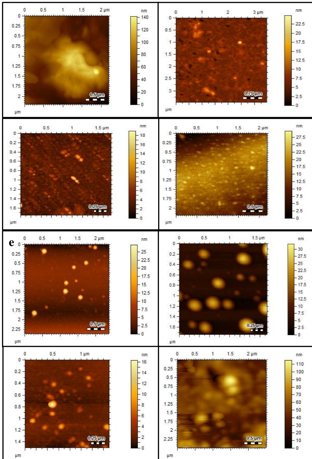
Gambar 8. Topografi 2 dimensi karbon dot a B-CDs1, b N-CDs1, c S-CDs1, d P-CDs, e B-CDs2, f N-CDs2, g S-CDs2, dan h P-CDs2
