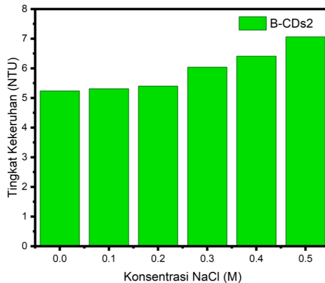
Gambar 16. Diagram tingkat kekeruhan karbon dot B-CDs2 terhadap variasi konsentrasi garam NaCl
