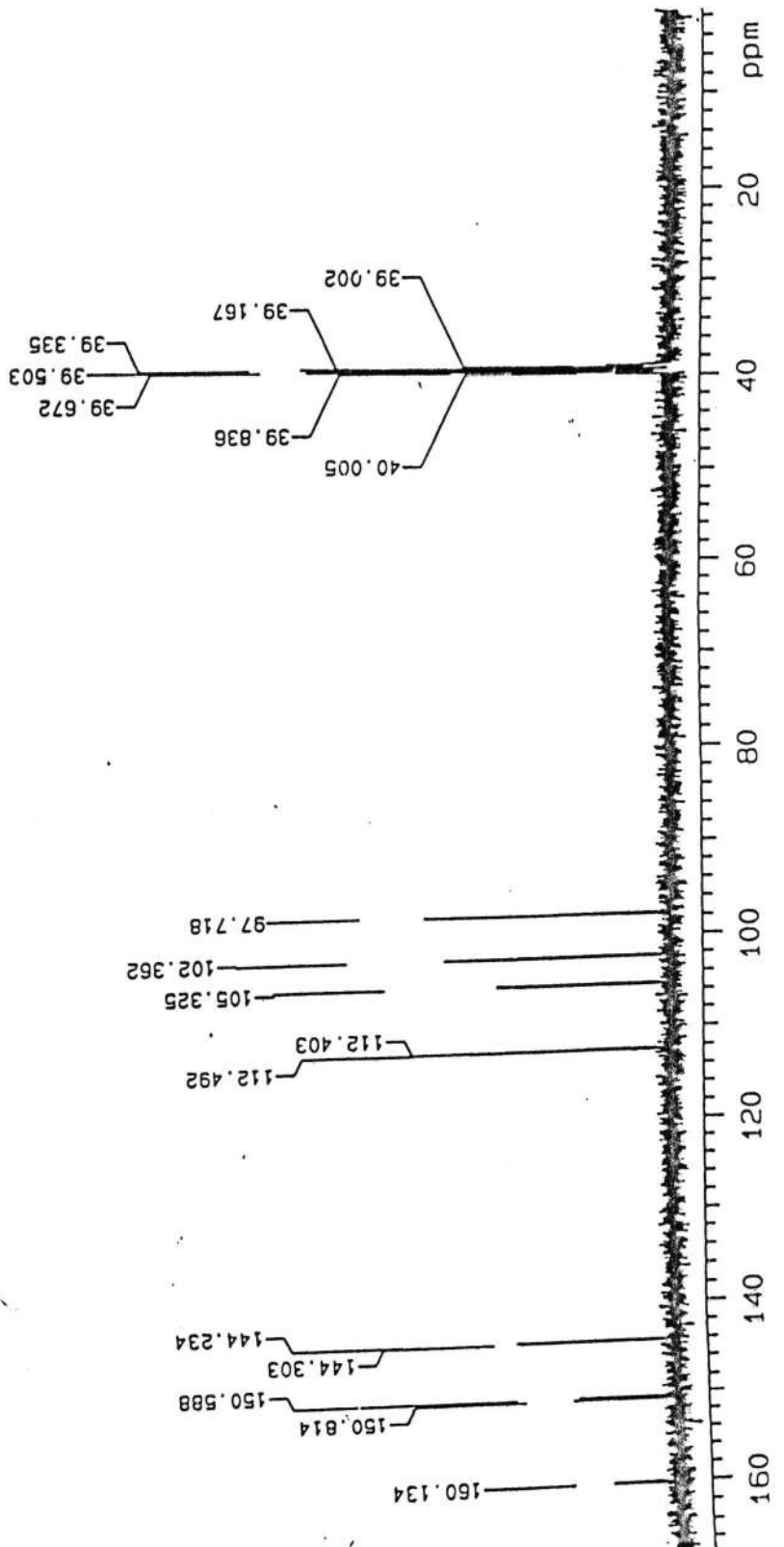
Spektrum ^{13}\text{C} -RMI (500 MHz) dalam \text{DMSO-d}_6 pada 40.0 C/313.1 K
