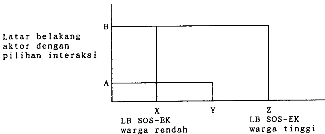
Gambar 5 Visualisasi Proposisi 4
