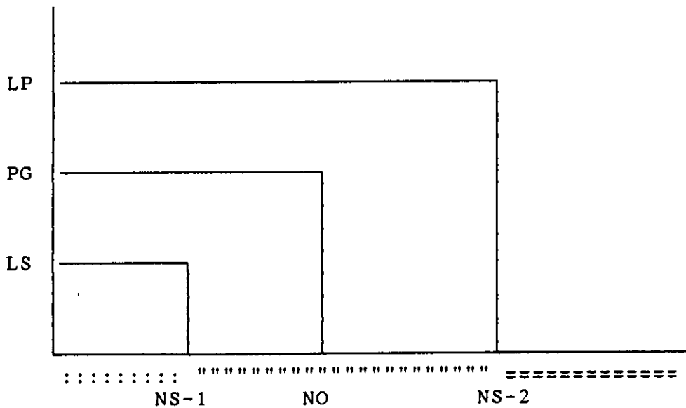
Gambar 3 Visualisasi Proposisi 1
