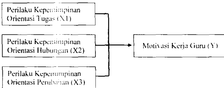
Gambar 3.1 Kerangka Konseptual
