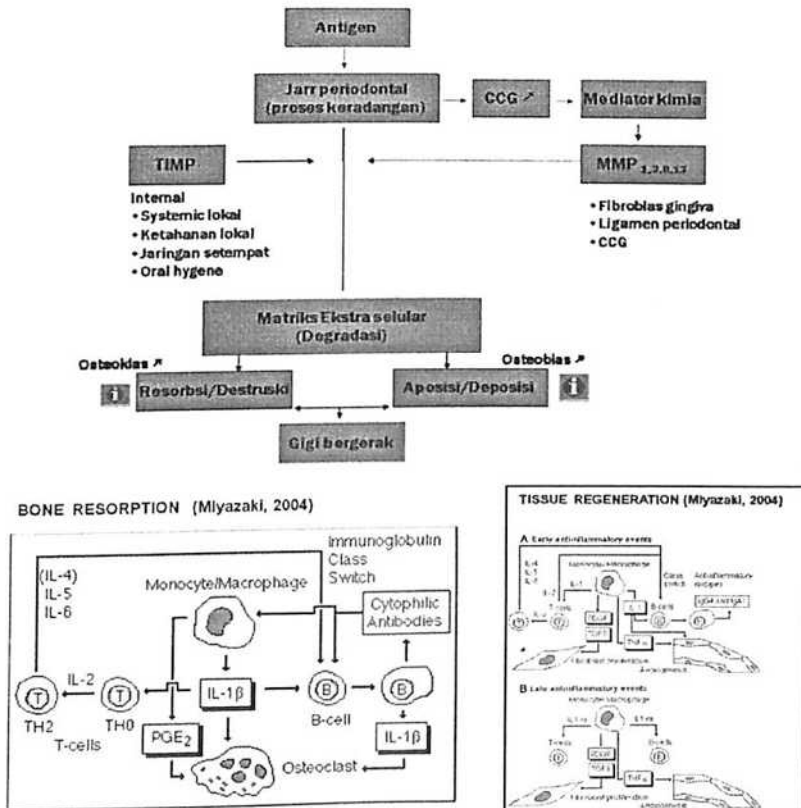
Gambar 1. Proses pergerakan gigi ortodonsi
