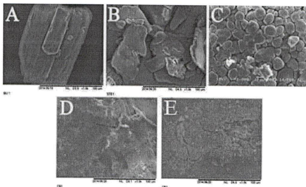
Gambar 5. Fotomikrograf SEM pada perbesaran 1000 kali
