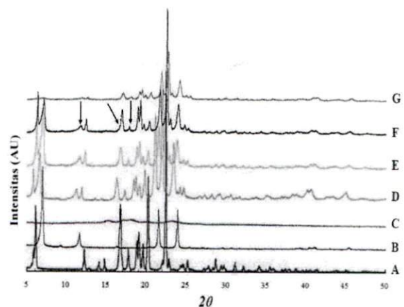
Gambar 2. Profil difraksi sinar-X serbuk
