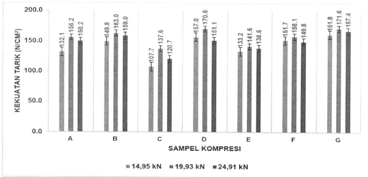
Gambar 1. Nilai kekuatan tarik
