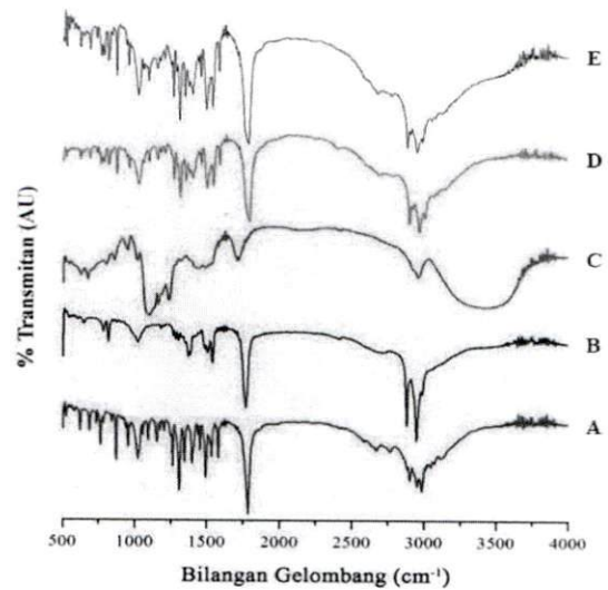
Gambar 4. Spektra inframerah
