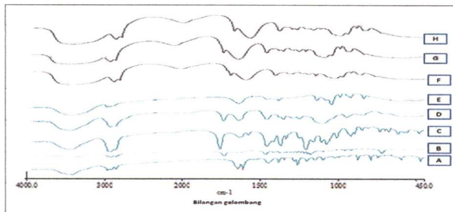
Fig. 2: Fourier transforms infrared spectrum of (a) coenzyme Q10; (b) Cetyl palmitate; (c) alpha tocopherol acetate; (d) Tween 80; (e) propyleneglycol; (f) F1; (g) F2; (h) F3
