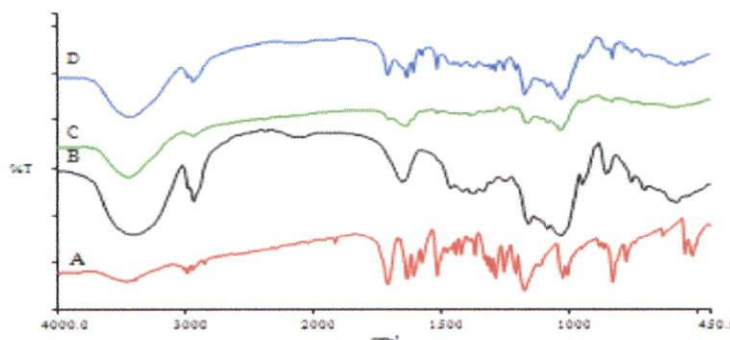
Fig. 3. FTIR spectra of EPMS (A), HP-β-CD (B), KI (C), CF (D)
