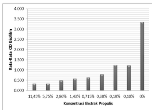
Gambar 2. Grafik Hasil Pengukuran ELISA Reader OD Biofilm
