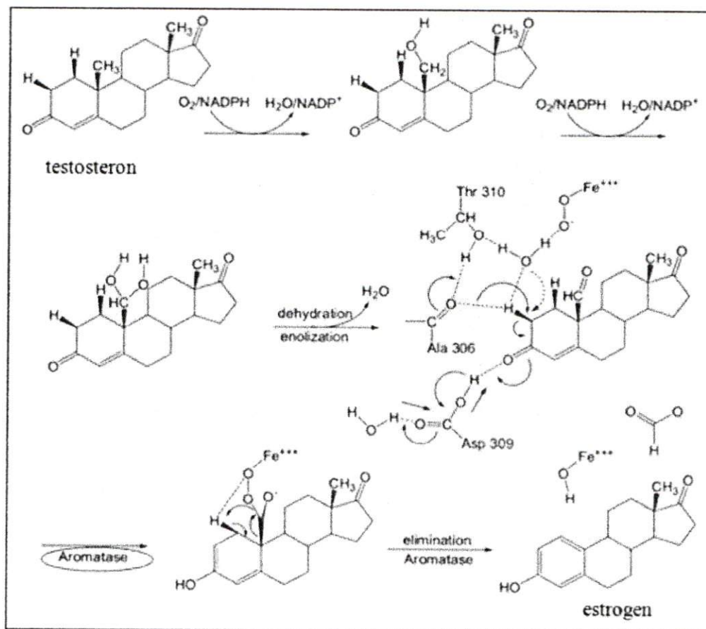
Gambar 5. Peran aromatase dalam mengubah hormon testosteron menjadi hormon estrogen (Suvannang et al. , 2011)
