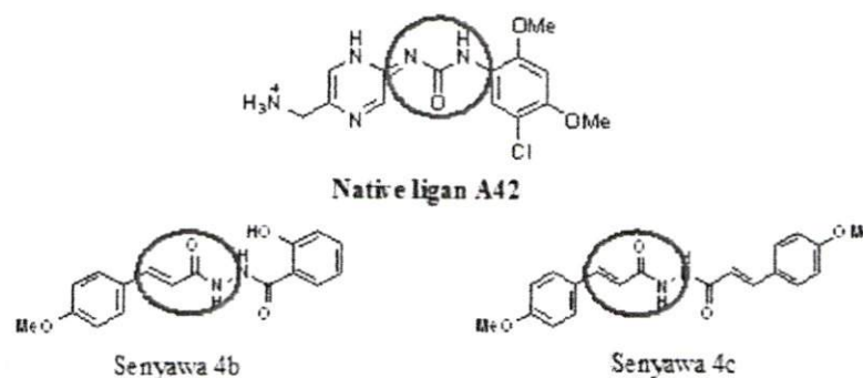
Gambar 9. Persamaan Struktur farmakofor native ligand A42 dengan senyawa 4b dan 4c
