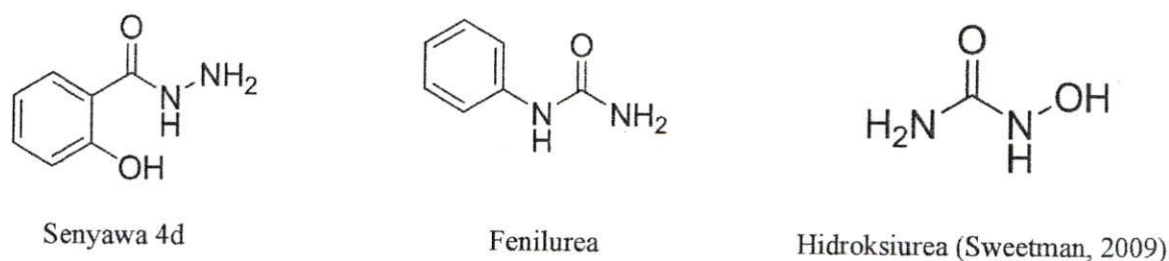
Gambar 3. Kemiripan struktur dalam menghambat enzim check point kinase 1
