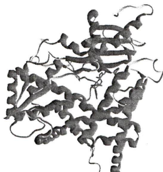
Enzim Aromatase (3S7S)
