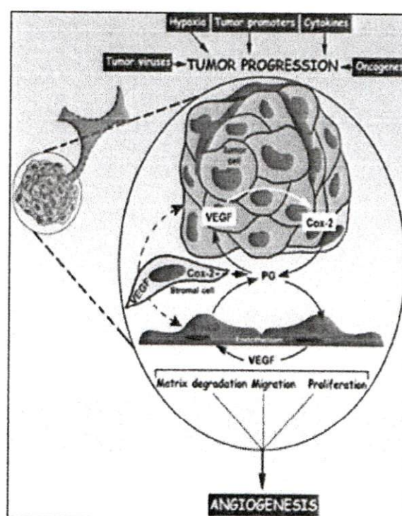
Gambar 1. Peran COX-2 pada proses angiogenesis (Iniguez et al. , 2003)
