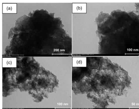
Fig 10. TEM images of AMA-72.
